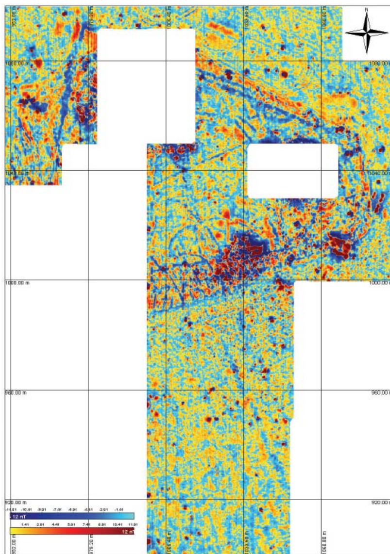
Figura 3. Sobari. Planul magnetometric al suprafeței investigate în campania anului 2009
