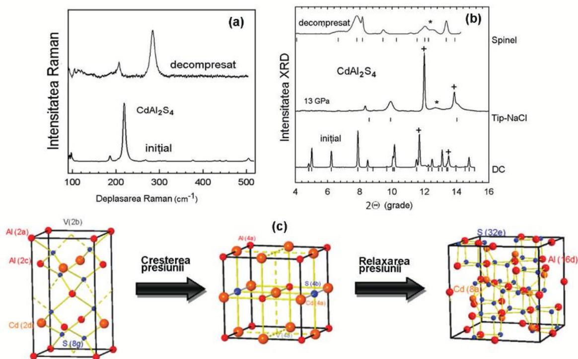
Figura 7. (a) Spectrul Raman al cristalului CdAl 2 S 4 inițial și cel de după decompresie. (b) Difractograma XRD a cristalului CdAl 2 S 4 inițial, după tranziția de fază în structura de tip NaCl și după decompresie. (c) Ilustrarea tranzițiilor de fază la compresie și la decompresie.
