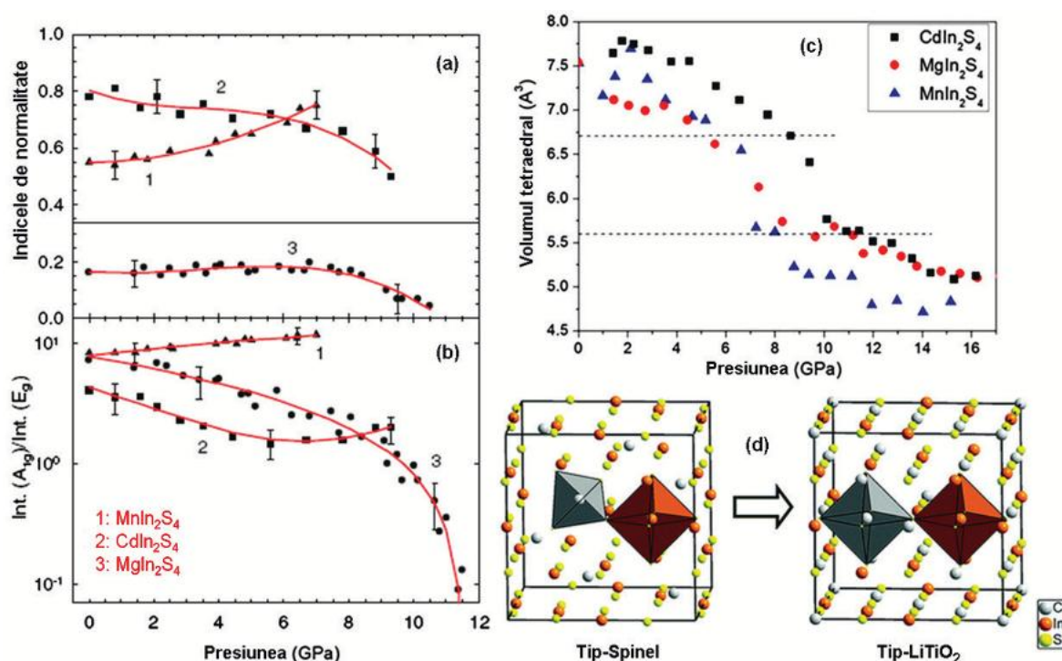
Figura 8. (a) Dependența de presiune a indicelui de normalitate în compușii A\text{In}_2\text{S}_4 . (b) Intensitatea integrală a modului A_{1g} normalizat la intensitatea modului E_g . (c) Evoluția volumului tetraedrelor în structura spinel la creșterea presiunii hidrostatice. (d) Ilustrarea tranziției de fază la compresie a compușilor A\text{In}_2\text{S}_4 cu structura inițială spinel.
