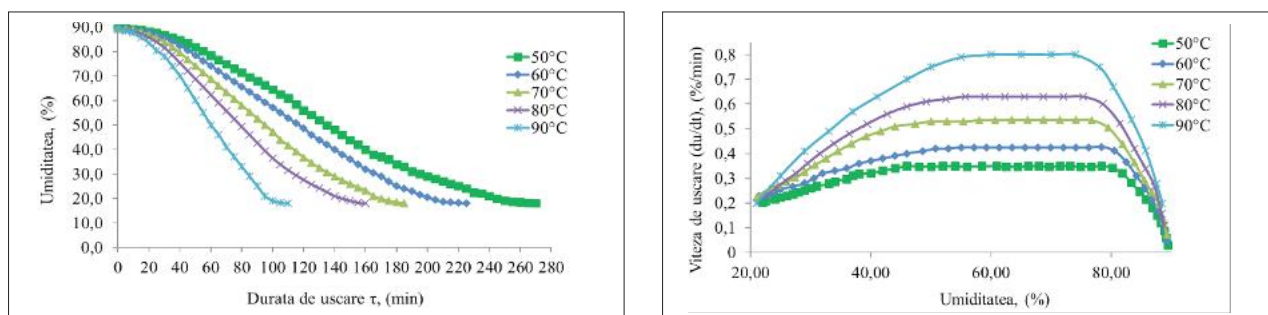
Figura 2. Cinetica deshidratării piersicilor la diferite temperaturi ale aerului – de 50-90 °C, viteză 2,0 m/s, umiditatea agentului termic 65 %, grosimea rondelui 4 mm.
