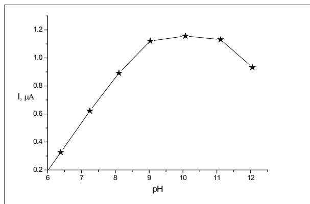
Figura 5. Dependenta curențului de reducere a ionilor de cadmiu cu ionii de magneziu din CdDCTA^{2-} în soluțiile de 5 mol/L NH_3 + 1 mol/L NH_4I de pH, C_{Mg} = 6 \cdot 10^{-5} mol/L.
