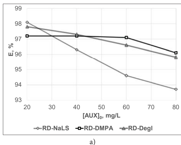
Figura 2. Performanța de înlăturare (%) rezultată la electroflotare (a) și electroflotare/coagulare (b); [RD]_0 = 200 mg/L, [Al^{3+}]_0 = 2,16 mg/L, pH=5,0-5,5, i = 0,5 Am -2 , t=10 min, V=0,25 L, t=25 °C.
