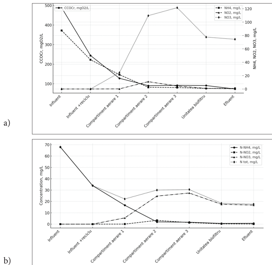
Figura 6. Diagrame: a) \text{CCO}_{\text{Cr}} , \text{NH}_4 , \text{NO}_3 , \text{NO}_2 ; b) N total, \text{N-NH}_4 , \text{N-NO}_3 , \text{N-NO}_2 ale proceselor simultane de nitrificare și denitrificare în fluxul tehnologic al stației de epurare a apelor uzate Căușeni la temperatura de 17,6 °C.
